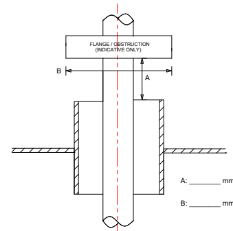
FLANGE ON PIPE / FLANGE OD
